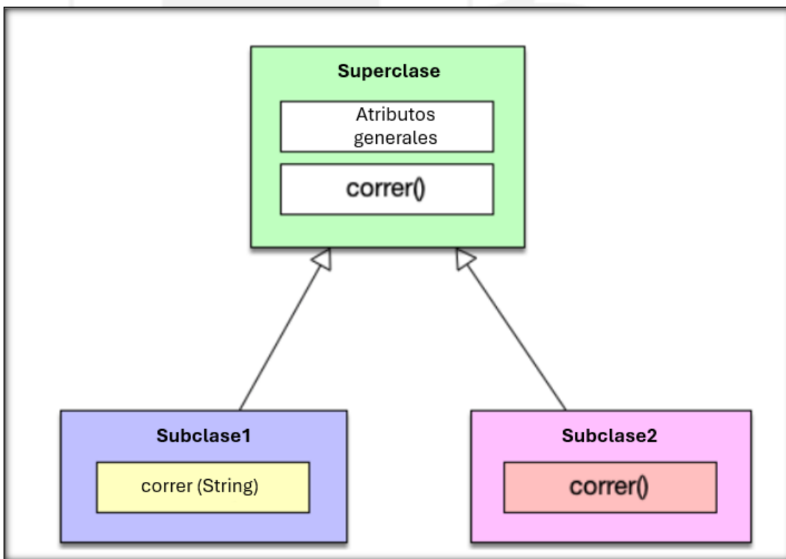
Ilustración 26: Visualización del Polimorfismo en Programación Orientada a Objetos
