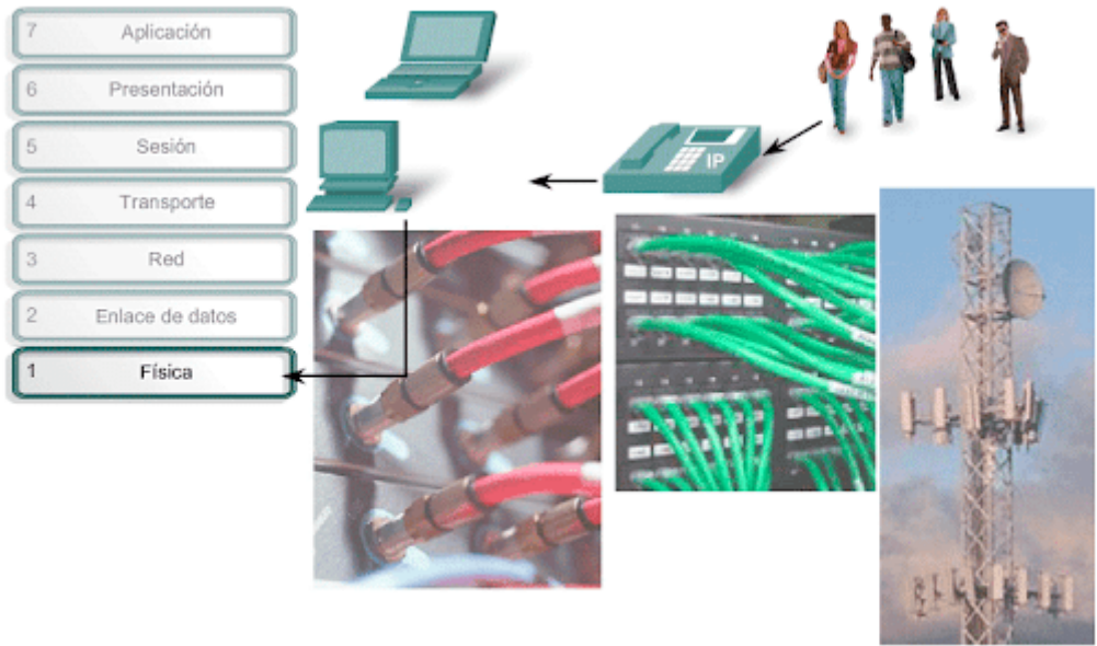
Ilustración 27: Capa Física
