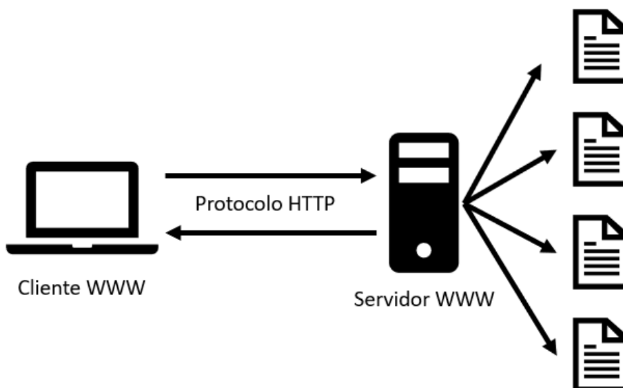
Ilustración 21: Protocolo HTTP
