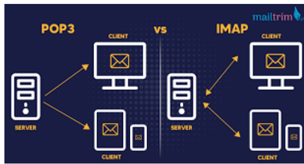
Ilustración 36: POP3
